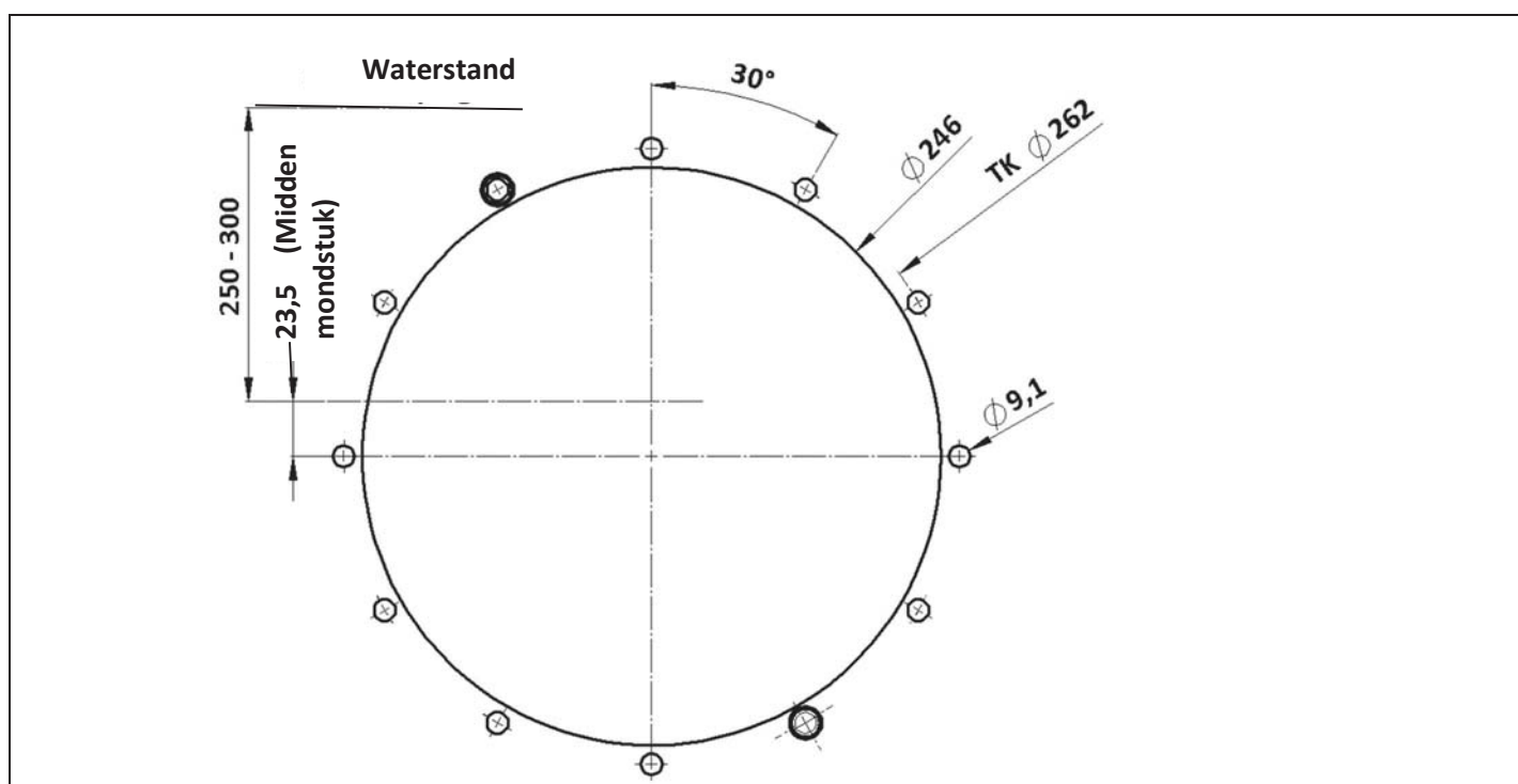
Afb. 10 Boorbeeld en bekkenuitsnijding afgewerkt bekken
