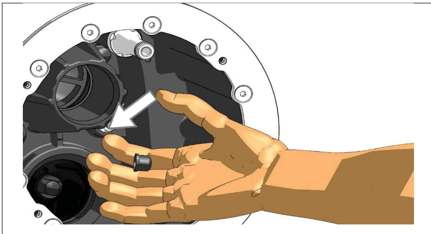
Afb. 20 De beschermingskappen op de zeskantmoeren drukken!
