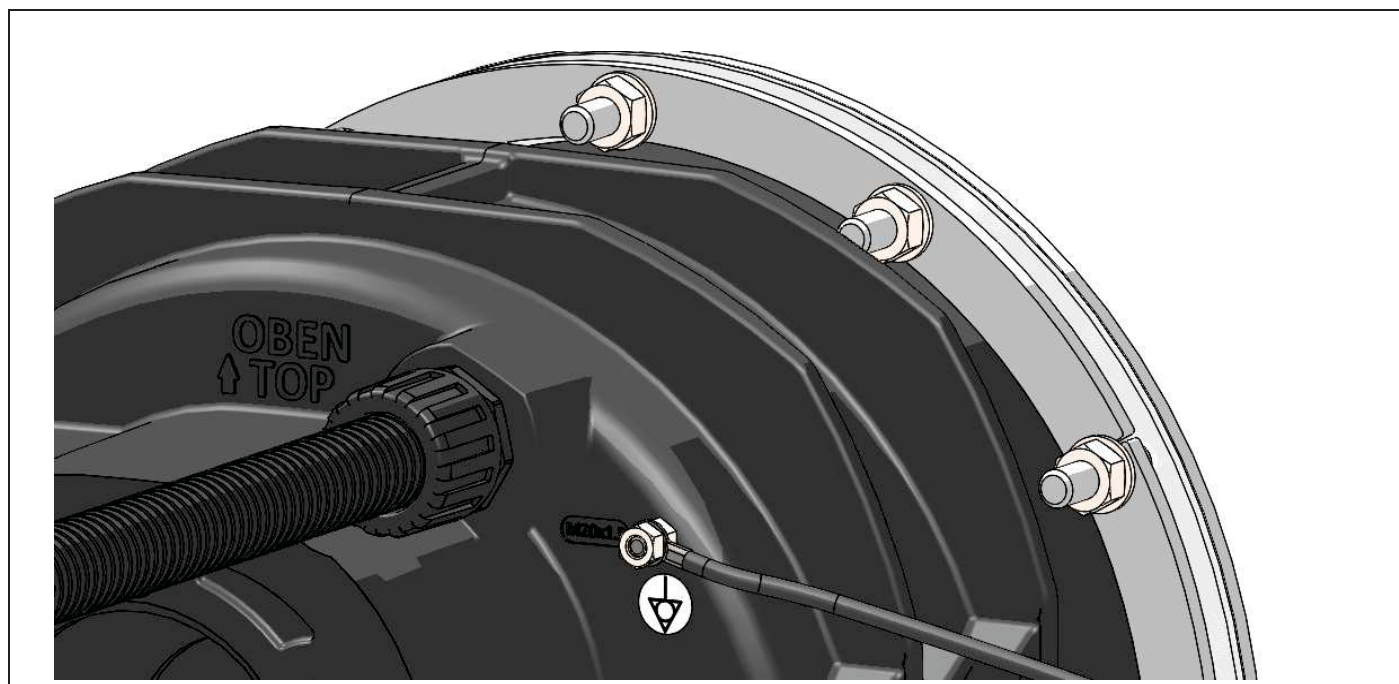
Afb. 1 Potentiaalcompensatiepunt inbouwbehuizing (voorbeeld PU)
