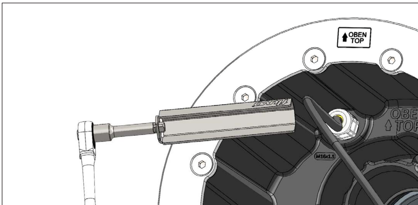
Afb. 24 Voor een eenvoudige montage het meegeleverde gereedschap gebruiken.
