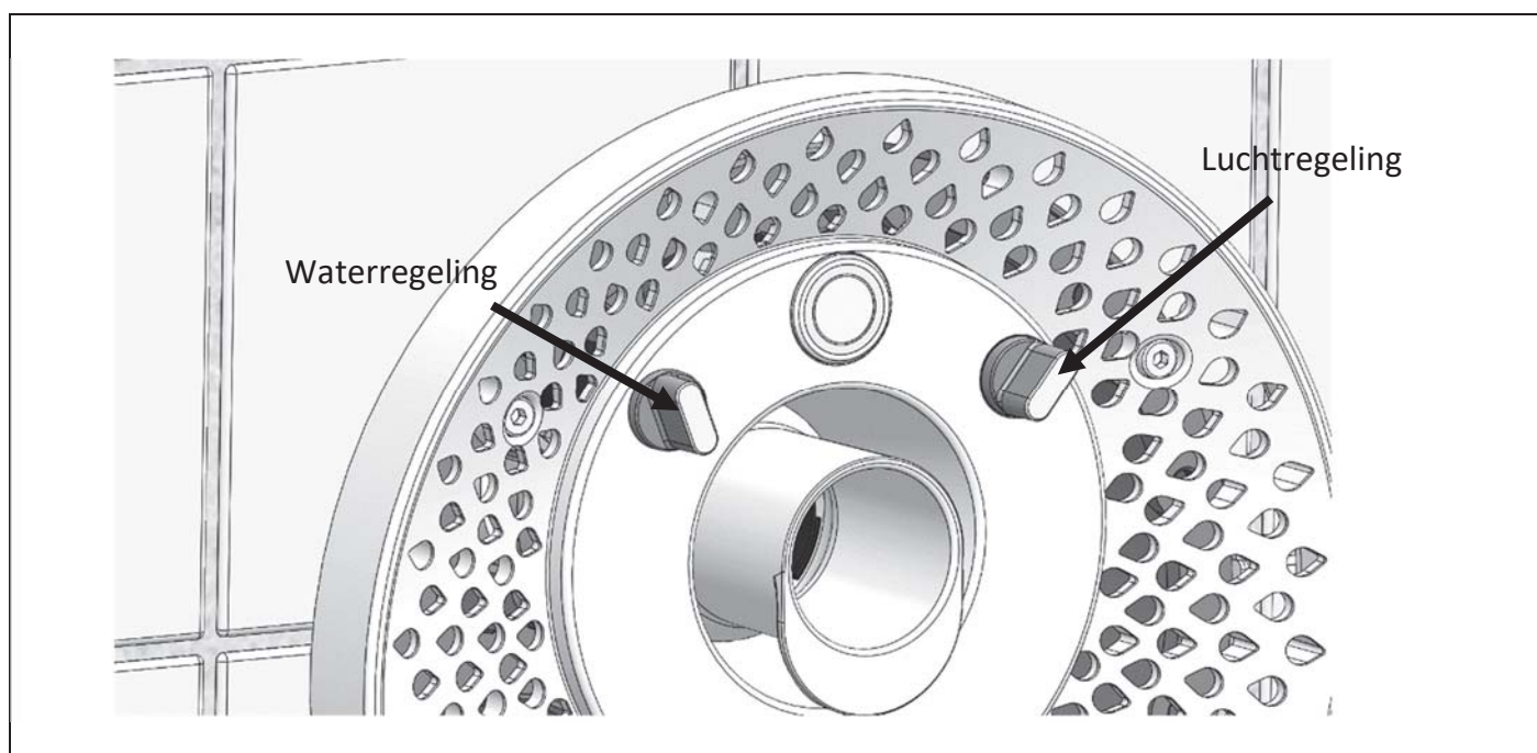
Afb. 34 Manuele regeling (draaigrepen voor de waterhoeveelheid en de luchttoevoer)
