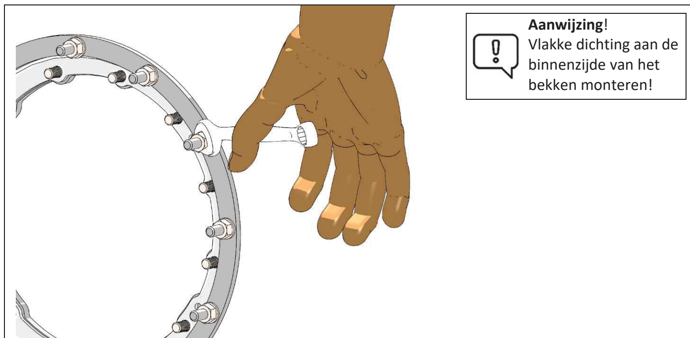
Abb. 14 Klemmring monteren
