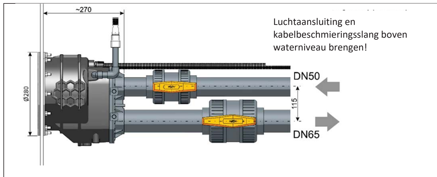
Afb. 4 Inbouwvoorstel gescheiden uitvoering (afbeelding uitvoering klaarbakken)
