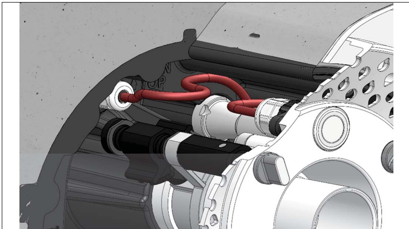
Afb. 23 Kabel (sensortoets) door kabelschroefverbinding trekken en aantrekken.
